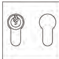
627.5 Profilzylinder, 61 mm, innen blind und außen mit Zylinder, 6 Stiftzuhaltungen mit Bohrschutz
