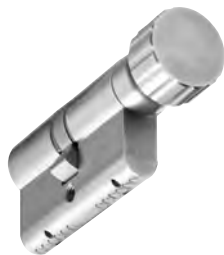
924 Profil-Knaufzylinder, 61 mm, 6+3 Stiftzuhaltungen einseitig und Knauf 22 mm Ø, mit Bohrschutz
