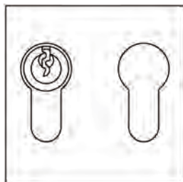
1527.5 Profilzylinder, 61 mm innen blind und außen mit Zylinder 5 Stiftzuhaltungen und 1 Flexcorenadel
