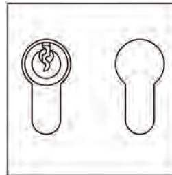
927.5 Profilzylinder, 61 mm, innen blind und außen mit Zylinder, 6+3 Stiftzuhaltungen mit Bohrschutz
