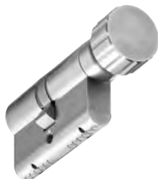
6524 Profil-Knaufzylinder, 61 mm, 6+5 Stiftzuhaltungen einseitig und Knauf 22 mm Ø, mit Bohrschutz
